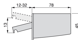
Sistema colgador a pared de módulos altos
