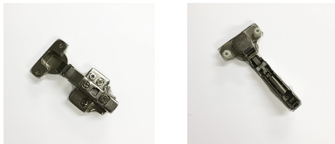
Bisagra de cazoleta con pistón amortiguador
